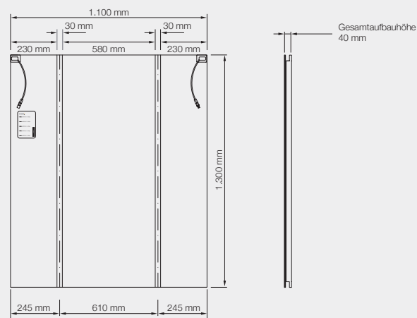
Rückansicht, Seitenansicht
